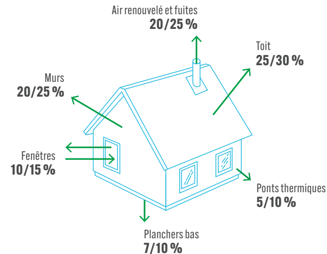
PERTES DE CHALEUR D'UNE MAISON CONSTRUITE AVANT 1974 ET NON ISOLÉE 1
